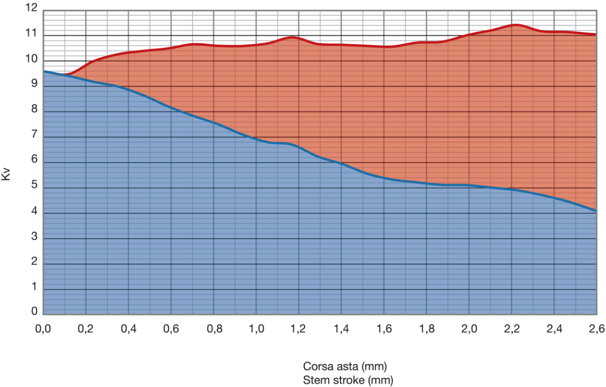
Diagramma primario/ricircolo con bypass aperto
